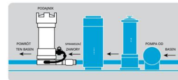
Ilustracja przedstawiająca podajnik Model 320
