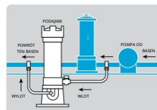
Ilustracja podajnika Model 300
